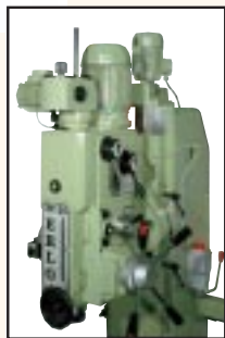
Sujeción neumática de la herramienta. Pneumatic clamping of the tool. Serrage automatique de l'outil. Pneumatisches Werkzeugspannen.
