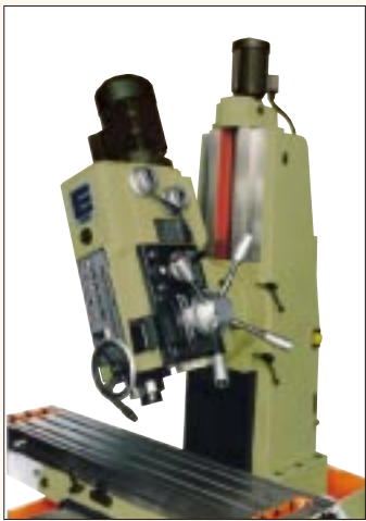
Cabezal basculante a cada lado del eje principal. Tilting head 45° both sides on main shaft. Tête basculante 45° a chaque côté del axe principal. Schwenkbarer Kopf auf 45° nach beiden Seiten der Hauptachse.
